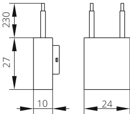
RC, DI suppressor
